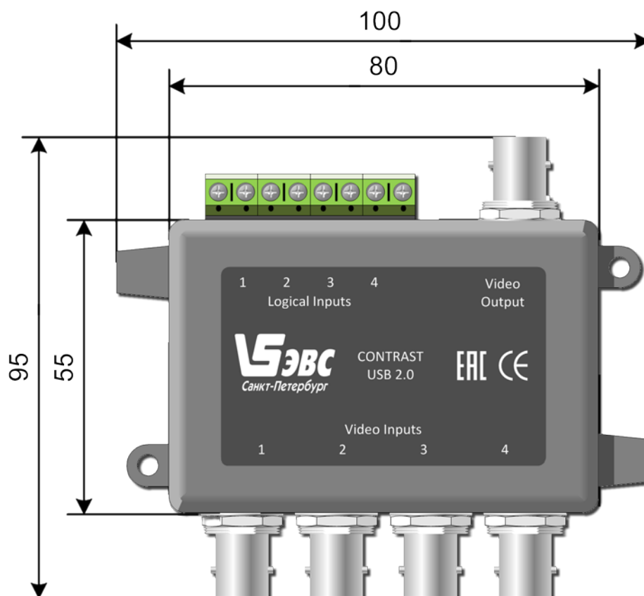
Рис.1. Устройство «Контраст-4-USB».
