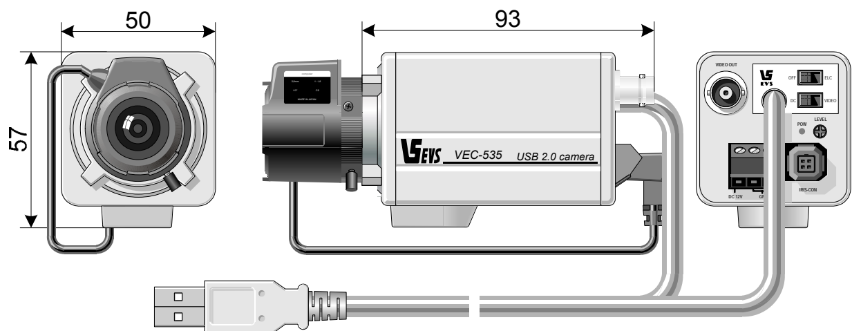
Рис.2. Камера VEC-535 .
