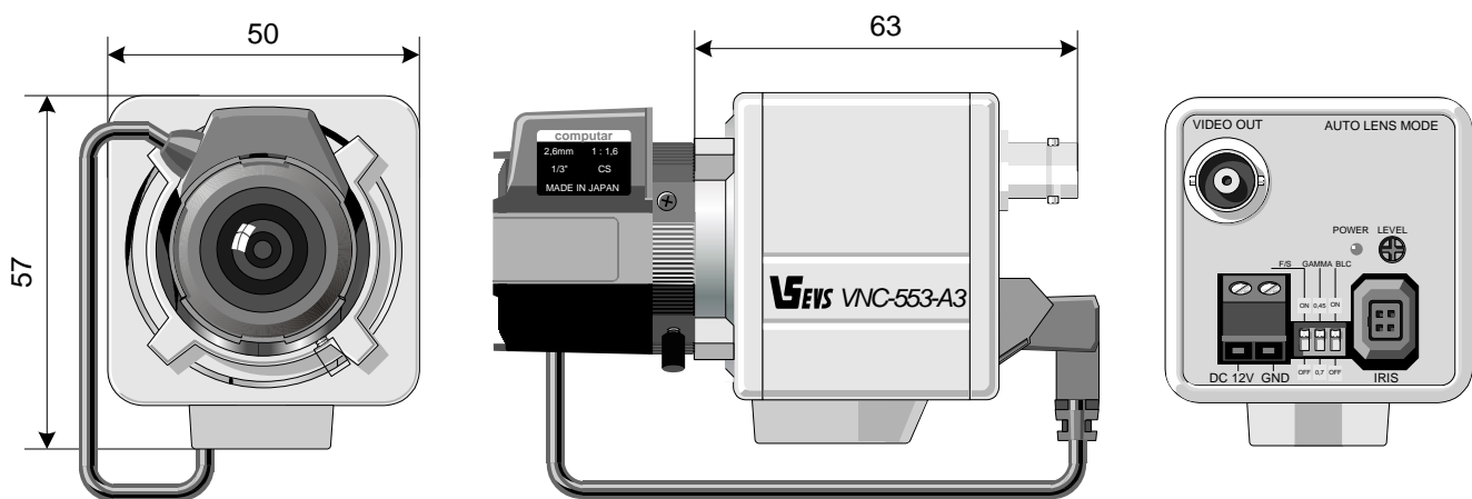
Рис.3. Камера VNC-553-A3
