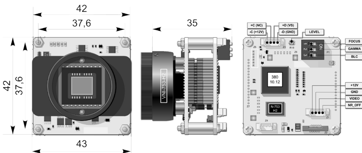
Рис.1. Камера VNI-753-H2
