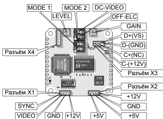
Рис.1. Камера VNN-743-A3. Внутренние органы управления и разъёмы камеры.
