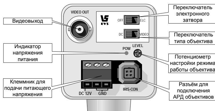
Рис.1. Камера VSC-541 . Органы регулировки и разъёмы для подключения питания, объектива и монитора.
