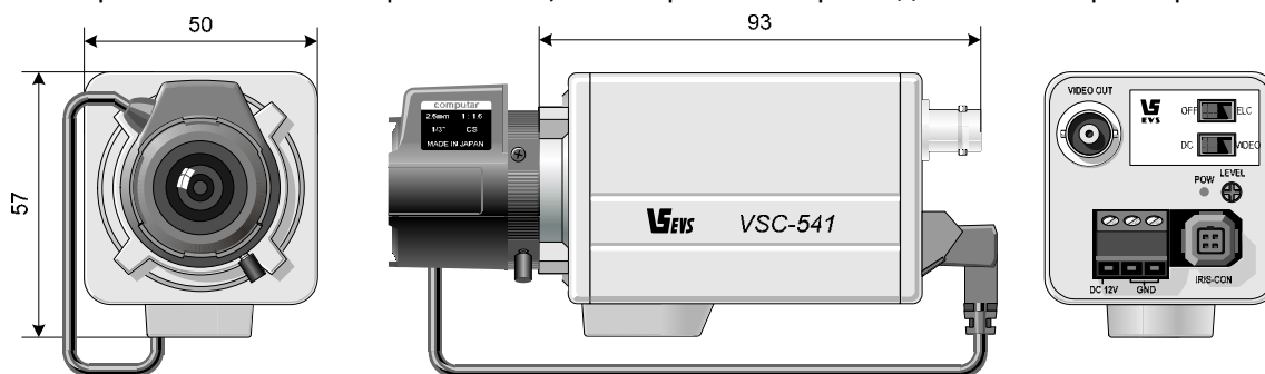
Рис.2. Камера VSC-541
