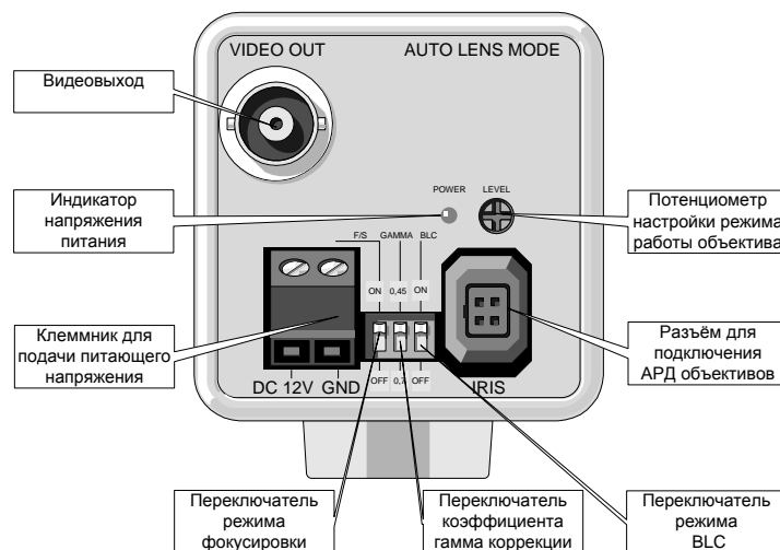
Рис.1. Камера VSC-551. Органы регулировки и разъёмы для подключения питания, объектива и монитора.
