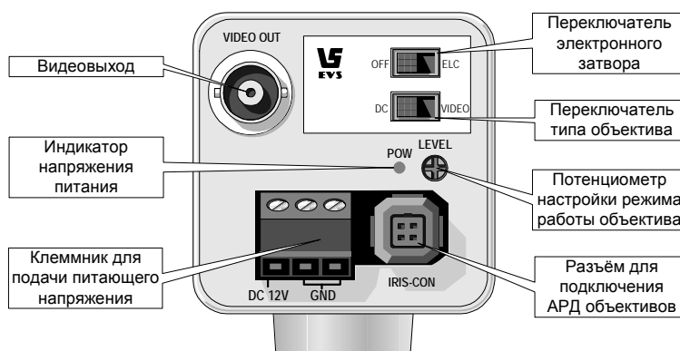
Рис.1. Камера VSC-746 . Органы регулировки и разъёмы для подключения питания, объектива и монитора.
