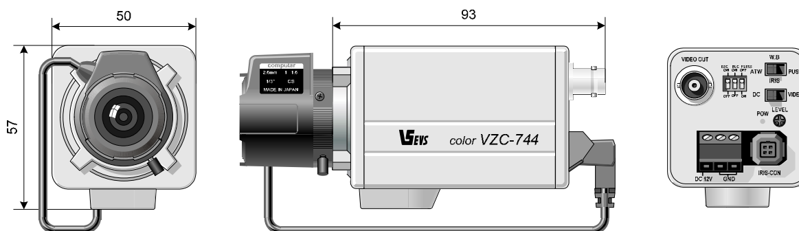
Рис.2. Камера VZC-744
