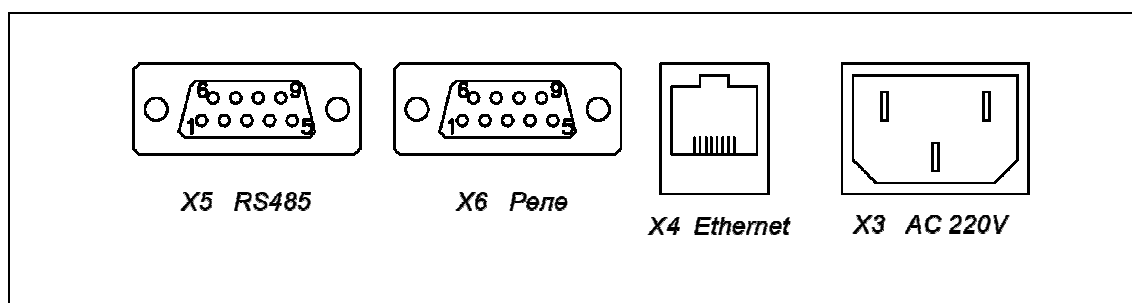
Рис. 3 Расположение соединителей для внешних подключений на верхнем торце секции управления.
