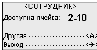
Рис. 42 Экранная форма доступа к ячейкам
