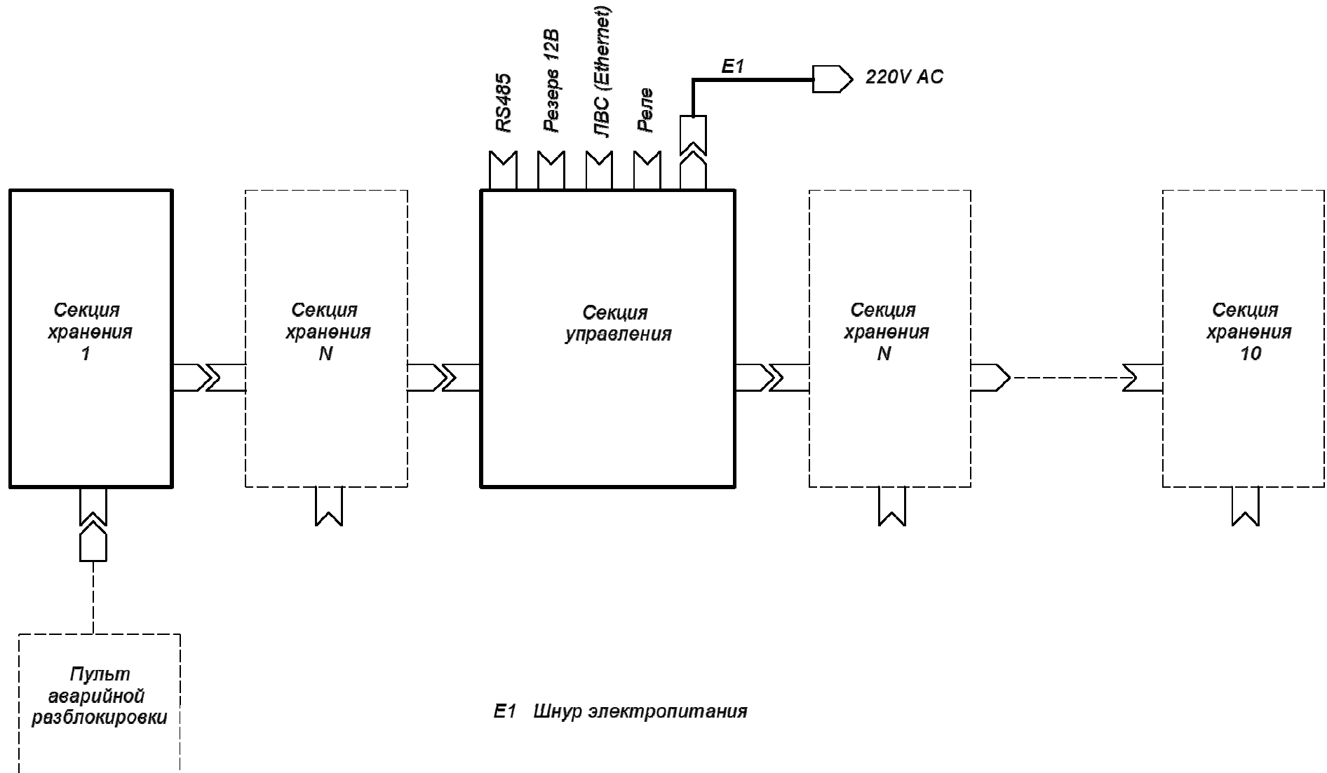
Рис. 41 Схема соединения секций изделия
