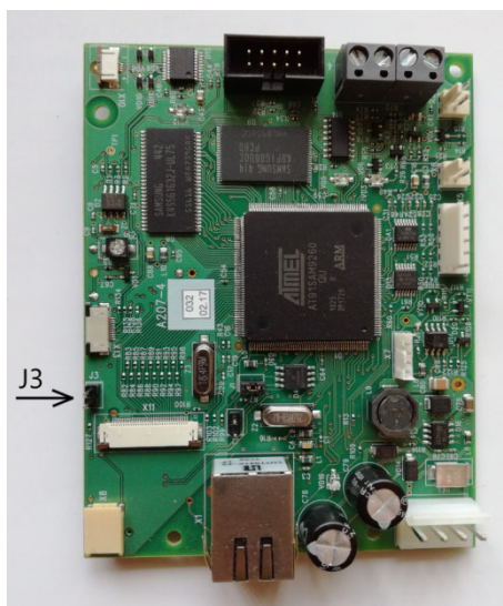
Рис. 39 Плата контроллера с указанием расположения джампера
